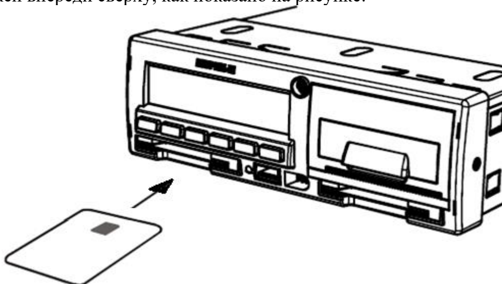
Рисунок 3 – Установка карты контролёра в слот «Основной водитель»
