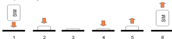
Рисунок 2 – Установка SIM-карты
