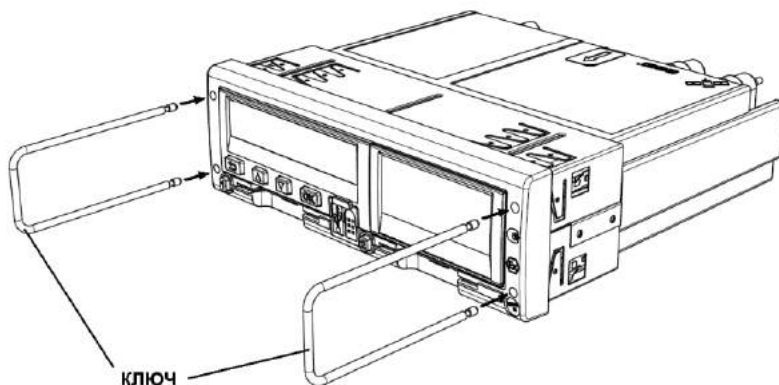
Рисунок 5 – Использование ключей для извлечения тахографа из кожуха.
