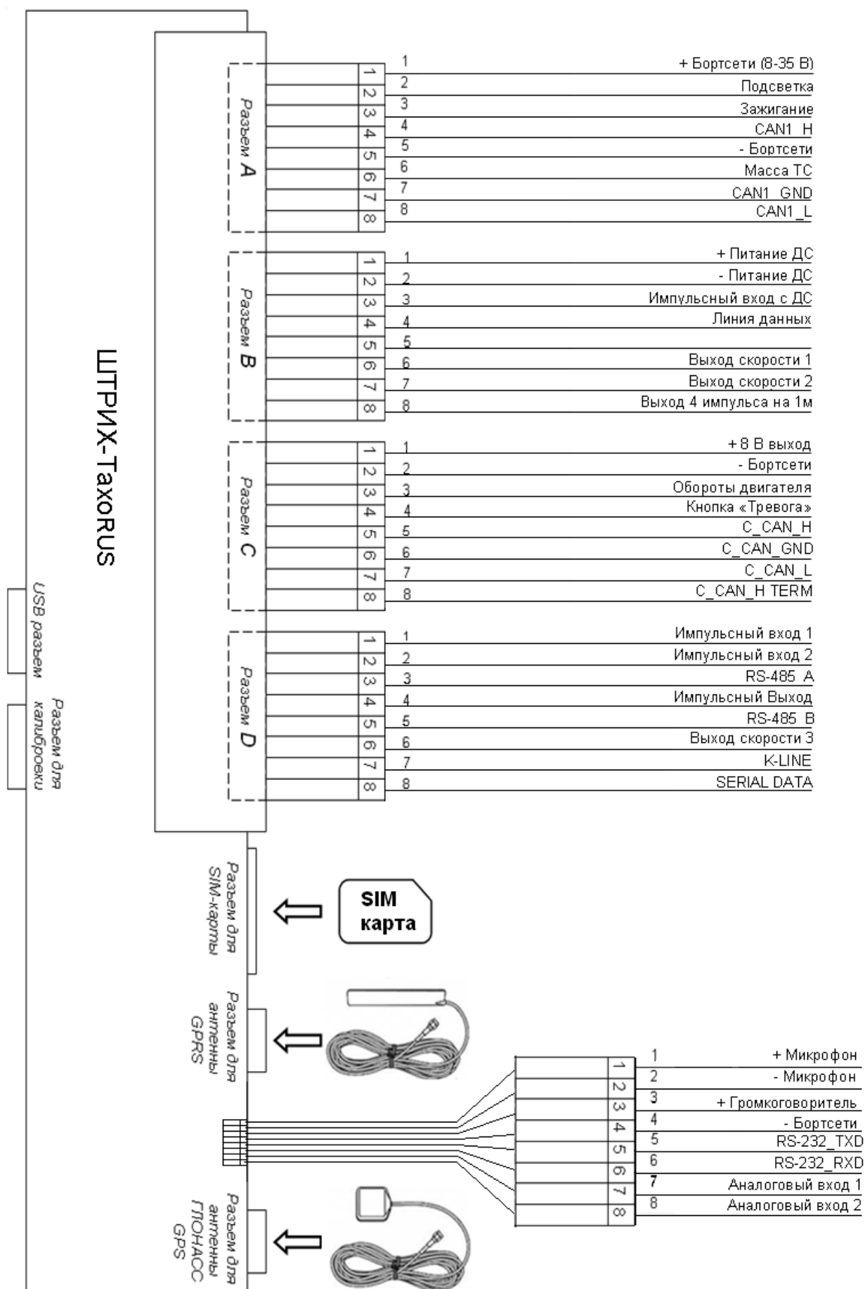
Рисунок 3 – Схема подключения тахографа «ШТРИХ – ТахоRUS»
