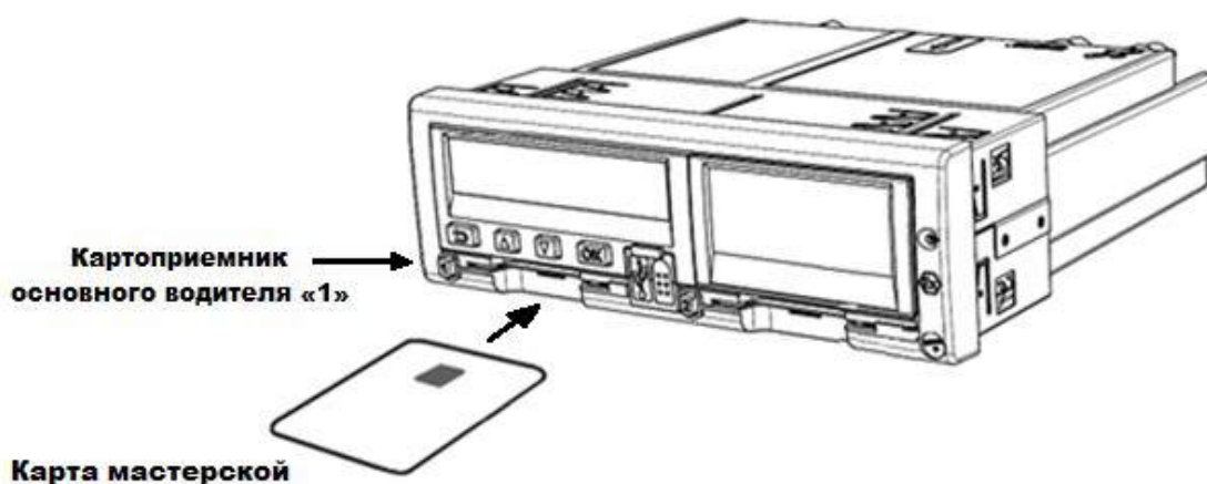
Рисунок 16 – Установка карты мастерской в картоприемник.
