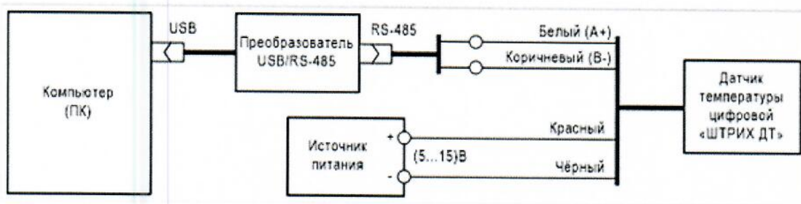
Рисунок 1 – схема подключения
